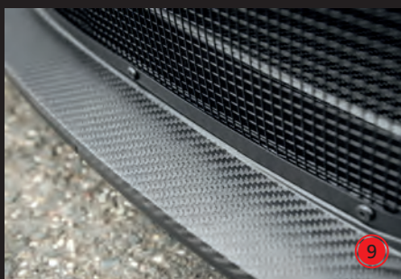
CARBON FRONTSPLITTER Frontsplitter inkl. steifigkeitsoptimierter Hauptträger und Skid Pads
